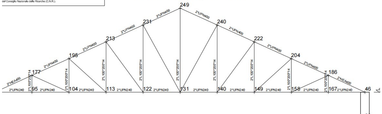
Schema telaio tipo (nodi 7-58-8)
